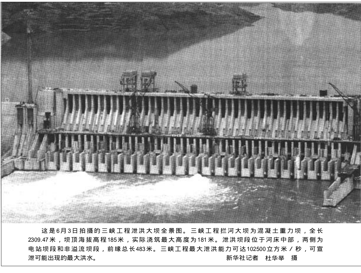
这是6月3日拍摄的三峡工程泄洪大坝全景图。三峡工程拦河大坝为混凝土重力坝，全长2309.47米，坝顶海拔高程185米，实际浇筑最大高度为181米。泄洪坝段位于河床中部，两侧为电站坝段和非溢流坝段，前缘总长483米。三峡工程最大泄洪能力可达102500立方米/秒，可宣泄可能出现的最大洪水。
